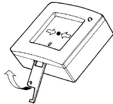
Fig. 2 - Apertura del pulsador
